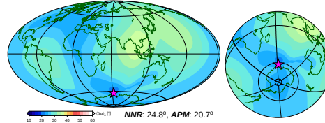
h) YB13 (63.4°, -62.7°, 0.271 °/Myr)
