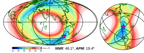
b) spr. align., Atlantic (130.4°, -50.1°, 0.625 °/Myr)
