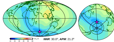
g) DR2012 (63.1°, -62.7°, 0.279 °/Myr)
