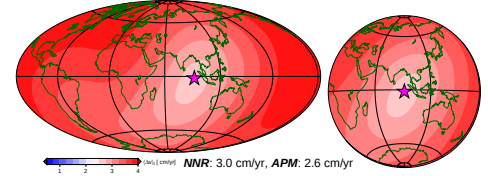
l) trench no mot. (91.6°, -1.9°, 0.200 °/Myr)
