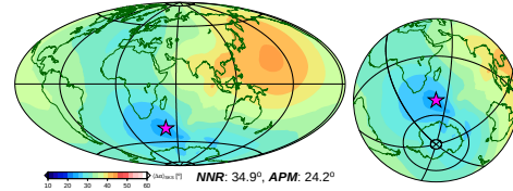
j) SKS-5 (45.7°, -45.2°, 0.252 °/Myr)
