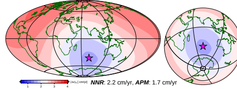
k) MM07 (79.4°, -41.9°, 0.166 °/Myr)
