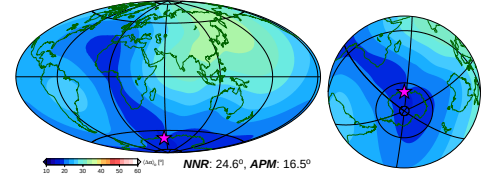
f) SL2013SVA (53.7°, -69.7°, 0.209 °/Myr)
